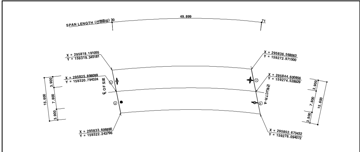
【그림 13.3.1】 교량받침 배치도
